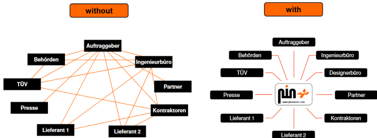
Abb. 1: Informationsfluss - Vergleich
